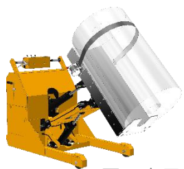
原反専用倒立搬送台車 (ロールピッカー-1)
