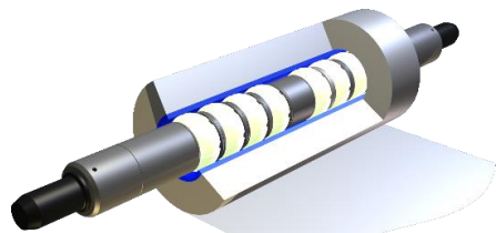
エアカプセル (エアシャフト)
