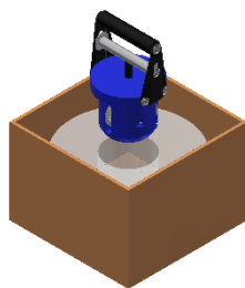
小型原反搬送治具 (ハンドキャッチャー)
